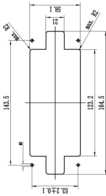
安装开孔图 Panel cut out
