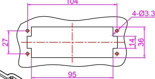
面板开孔图 Panel cut
